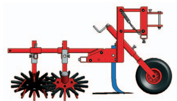
Hackmesser 1-teilig mit Fingerhacke
