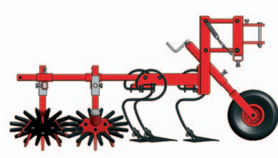
Hackmesser 3-teilig mit Fingerhacke
